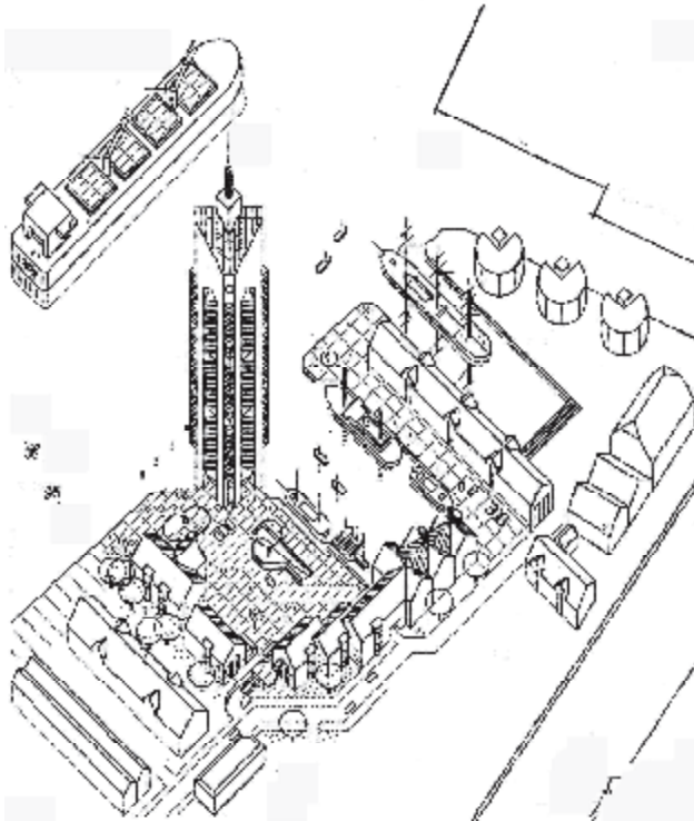
Godfred Louis Jensens forslag til byggeri på Krøyers Plads, et tårn med luft omkring
